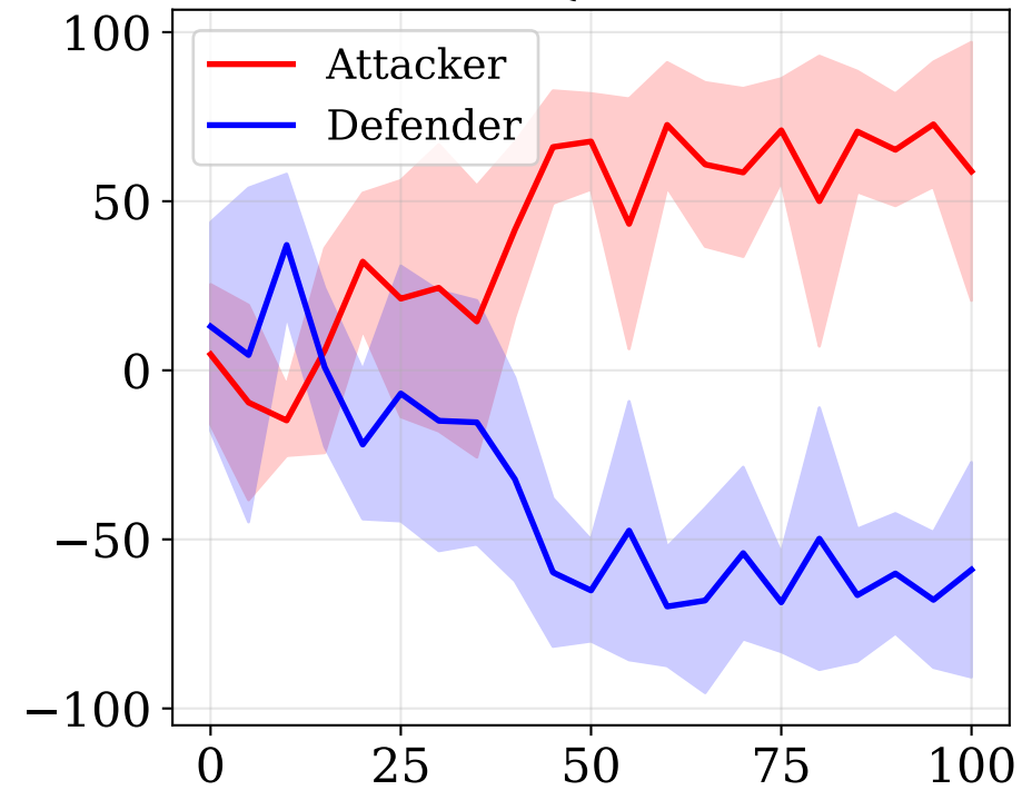
PPO Att vs DQN Def: Reward
